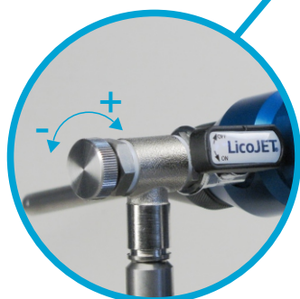
Flüssigkeitsmenge regulieren
